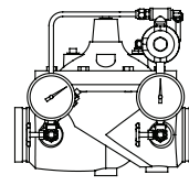
ZW209FPG Grooved Max 300 psi Inlet
