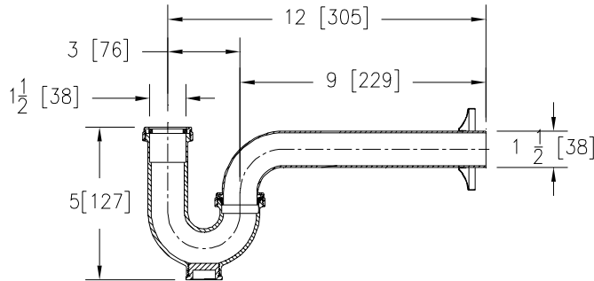
P-TRAP
